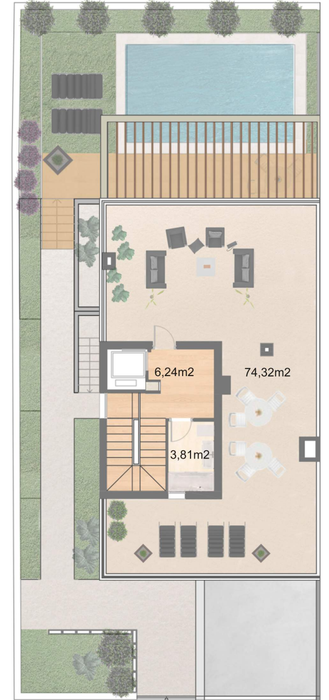
PLANTA SEGUNDA
