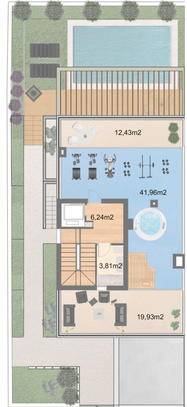
PLANTA SEGUNDA
