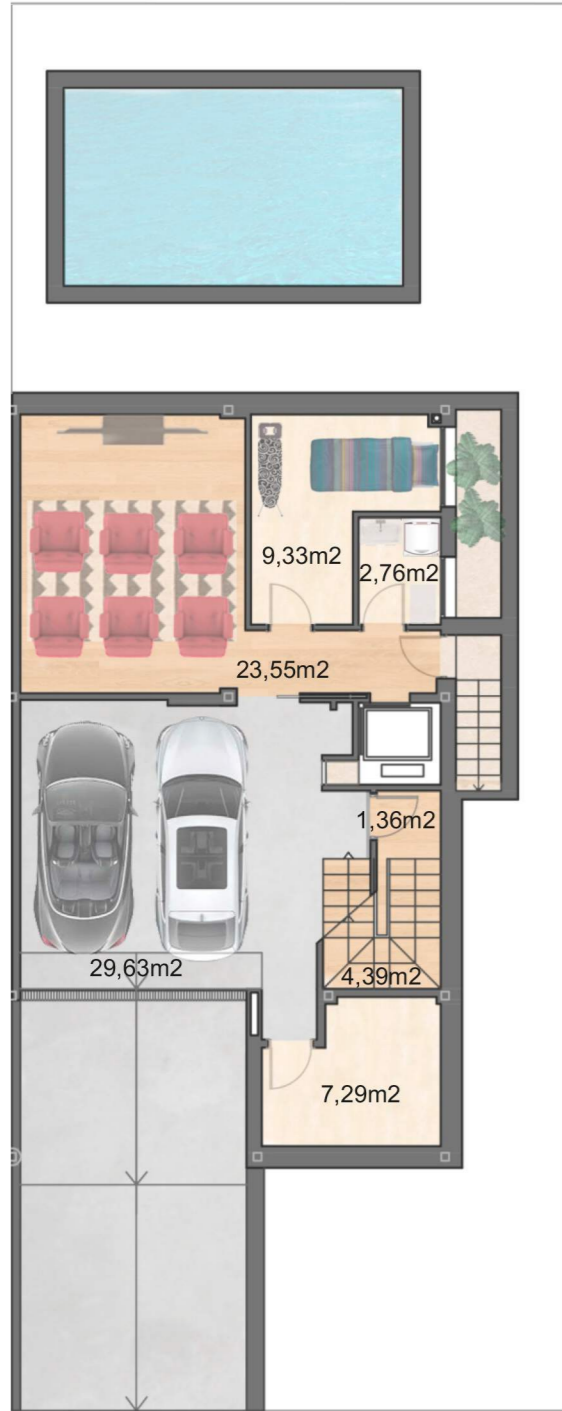
PLANTA SEMISÓTANO
