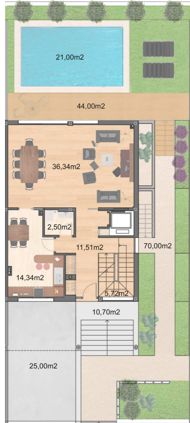
PLANTA BAJA
