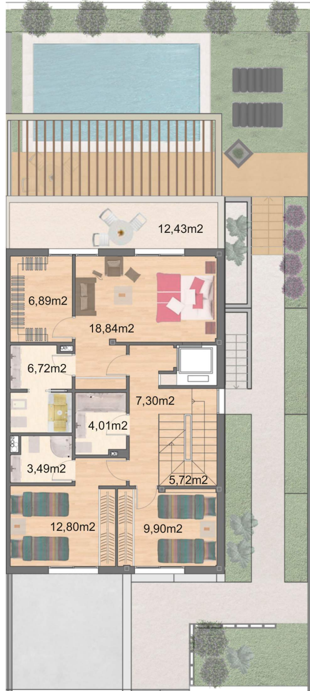
PLANTA PRIMERA
