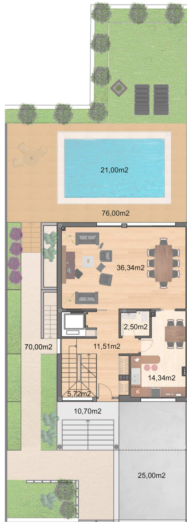
PLANTA BAJA
